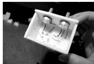
Fig. 1. Processo construtivo
